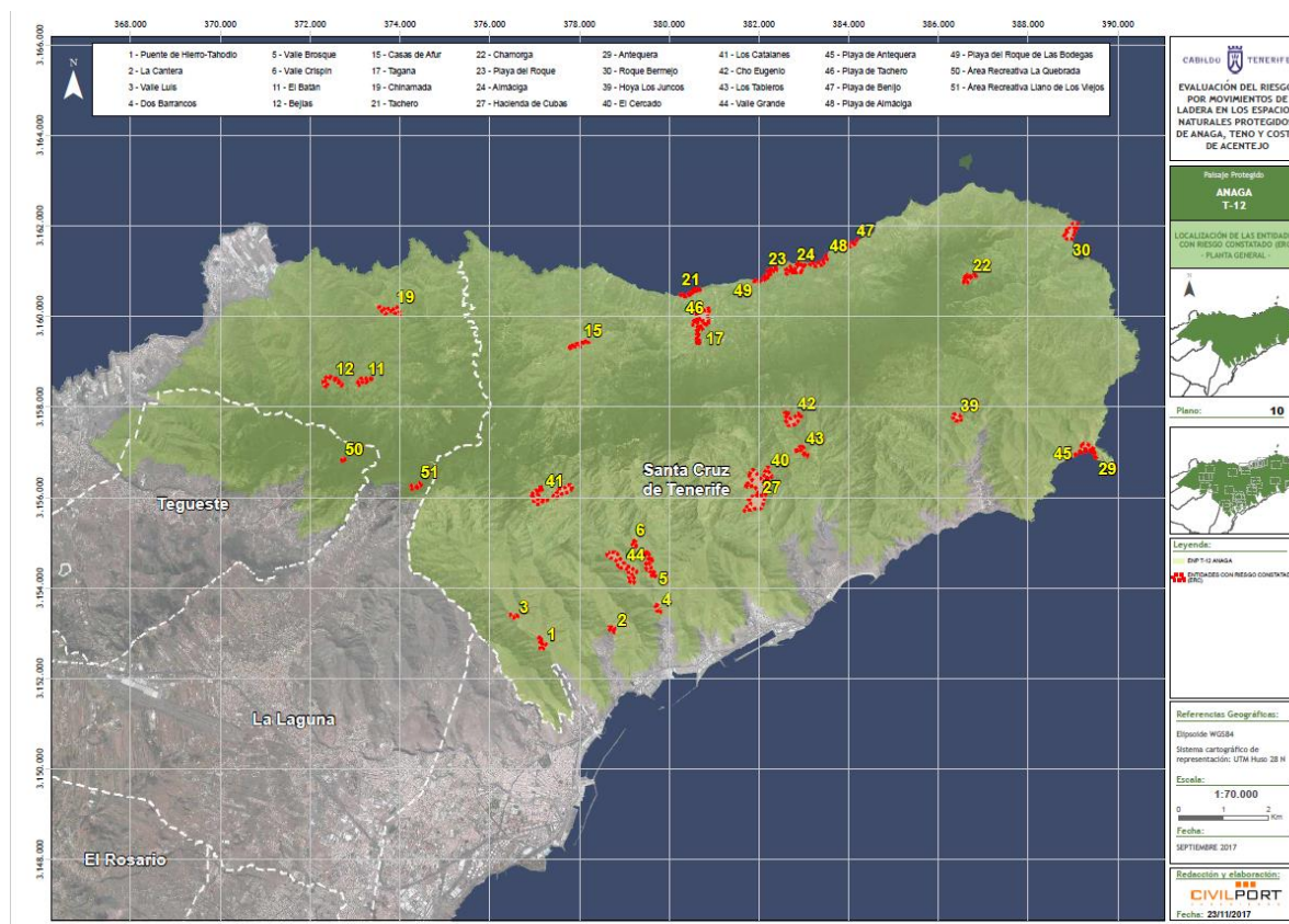
Mapa 7.- Localización de las entidades con riesgo constatado. Fuente: Estudio de riesgos por movimientos de ladera en el PR de Anaga (CivilPort Ingenieros, 2017)
